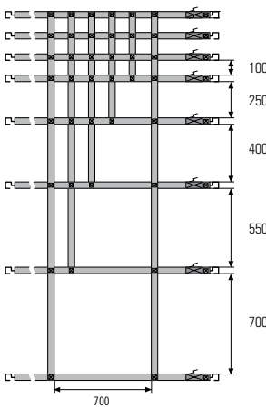
Lichte Maschenweite in mm für 50-mm-Gurtband
