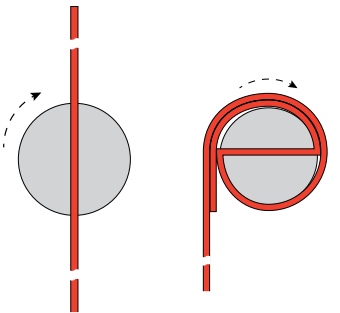
6 Aufwicklung des Gurtbandes bei der ST F -Prüfung
