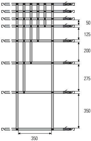
Lichte Maschenweite in mm für 25-mm-Gurtband
