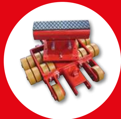
Sonderaufbau JLB 20 G
