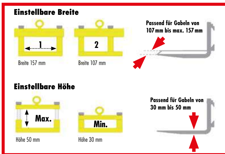
Ladungssicherung mit Gabelklemmen und Spanngurten.
