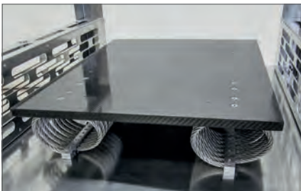
Aufnahmetisch, schwingend gelagert mit Gummipuffer oder Drahtseildämpfer
